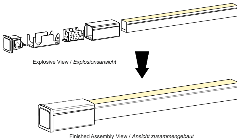
Finished Assembly View / Ansicht zusammengebaut
